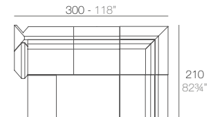
1 x 53004 Módulo Central - Sectional Sofa Armless 1 x 53002 Módulo Izquierdo - Sectional Sofa Left 1 x 53003 Módulo Derecho - Sectional Sofa Right 1 x 53005 Puff - Ottoman 1 x 54006 Módulo Esquina - Sectional Sofa Corner
